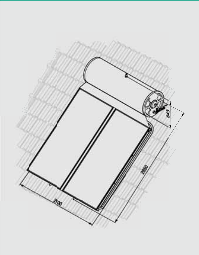
auroSTEP pro VTS 2-200 e VTS 2-300 su tetto inclinato
