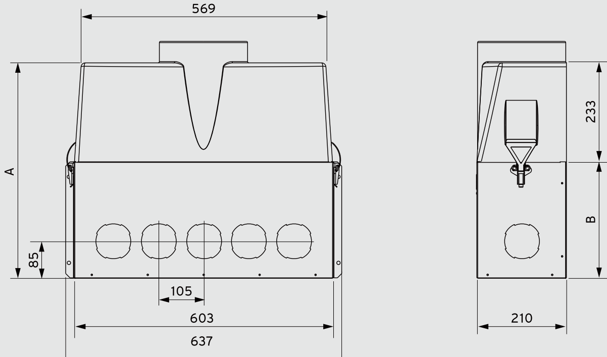
Diffusore/collettore d'aria (Misure in mm.)
