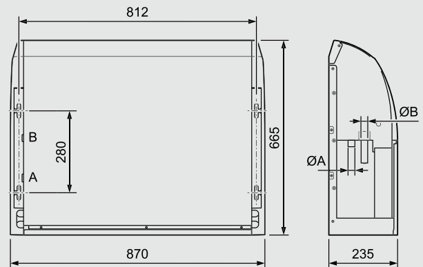
Vista posteriore
